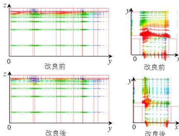
図1 鉄芯中の磁束分布の均一化 図2 鉄芯中振動の低減
